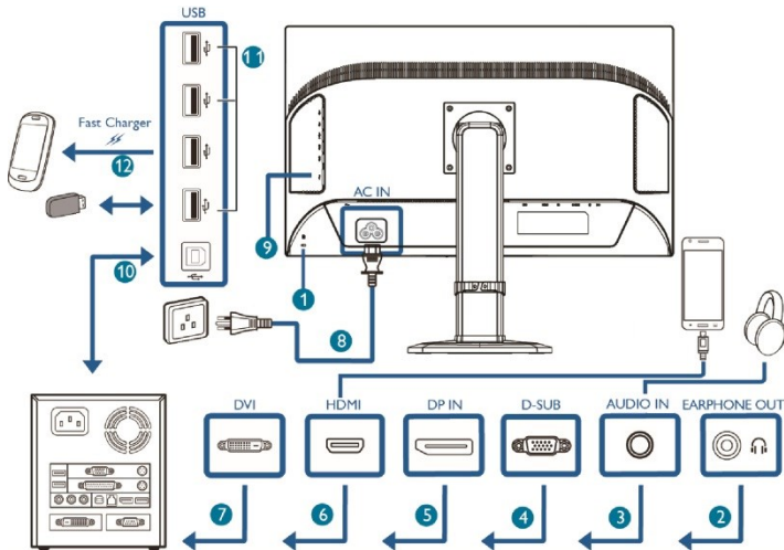
Figura 3 Conectar los cables
